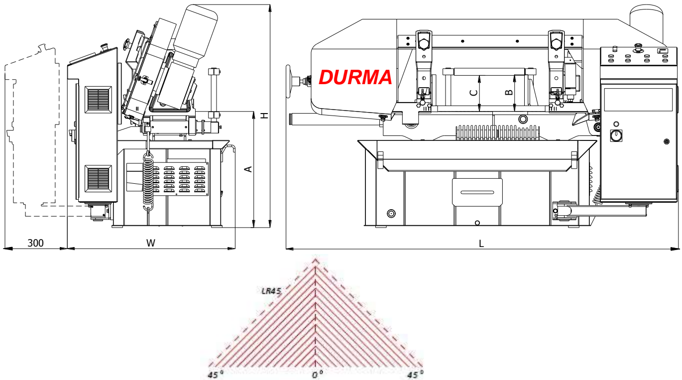
HB-S 330 (Kétoldali szögbevágó forgószámollyal)
